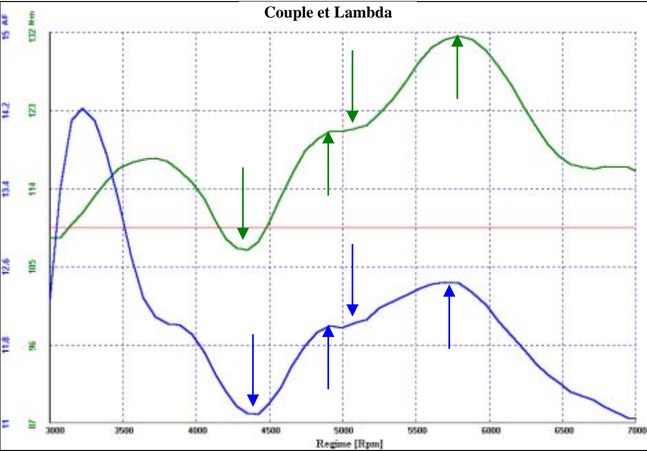
Haut correspondance valeurs Lambda et Couple
